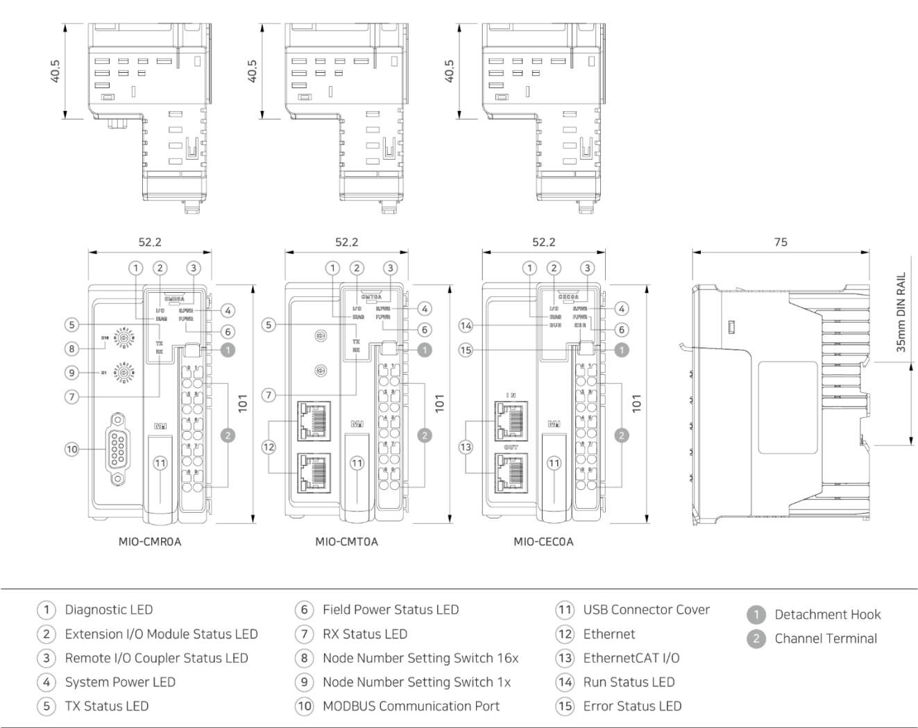
I/O MODULE
